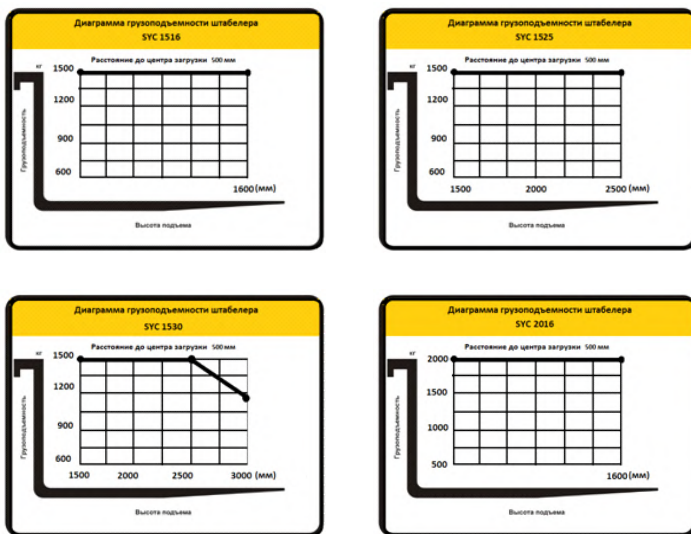
Рисунок. 4. Диаграмма грузоподъемности штабелера.
