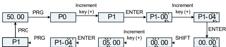
Рисунок 4-3 Блок-схема операций настройки параметров
