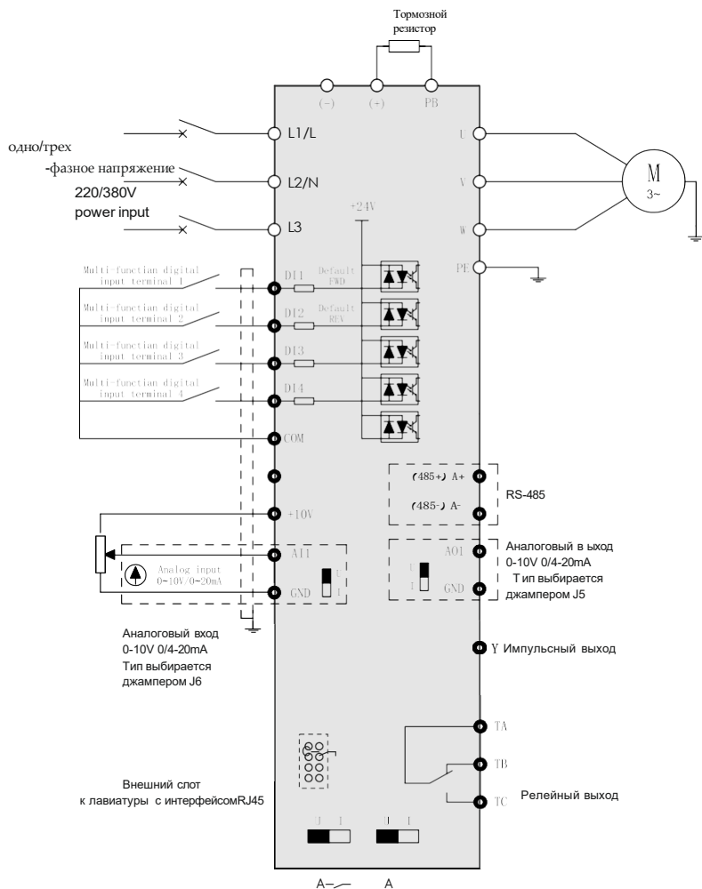
Рисунок 3-3 Схема подключения клемм
