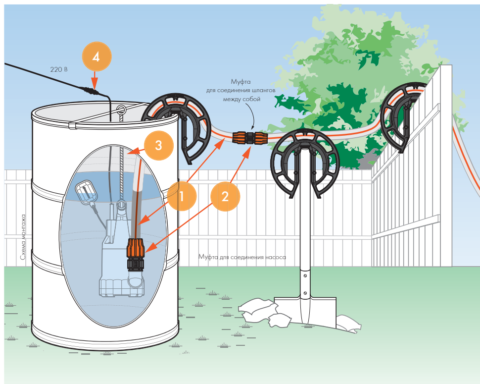
Рисунок 5. Пример монтажа насоса в емкости с применением шланга «УДАВ»
