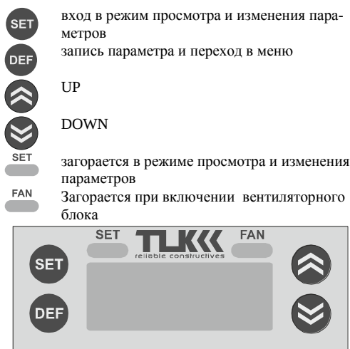
Передняя панель контроллера
