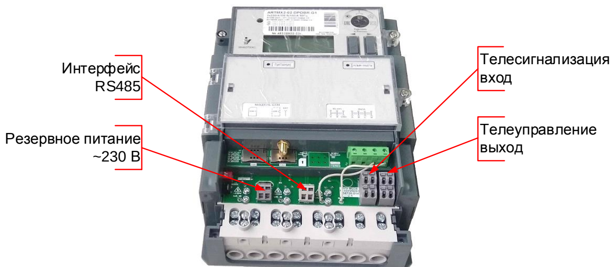
Рисунок 5.5 – Элементы подключения счетчика «Меркурий 234» с индексом «Х»
