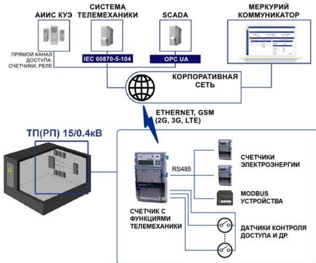
Рисунок 4.4 – Схема работы в составе автоматизированных систем
