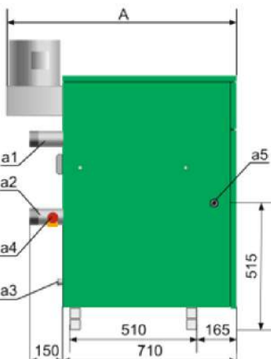
a3 Сливной патрубкок котла a4 Соединение предохранительного сбросного клапана
