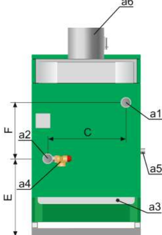
a5 Соединение для газопровода a6 Соединение для дымохода
