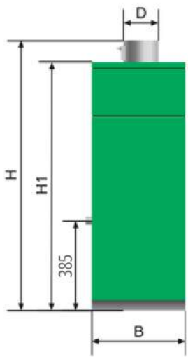
Размеры для Изнаир 30А 40А
