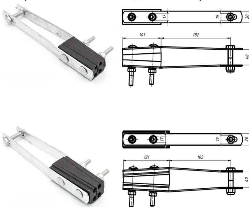
Рис. 1. Внешний вид анкерных зажимов RPA 425/50, RPA 425/120.
