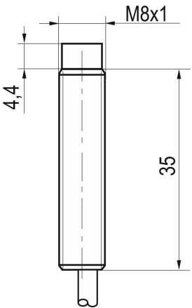
Габаритный чертеж
