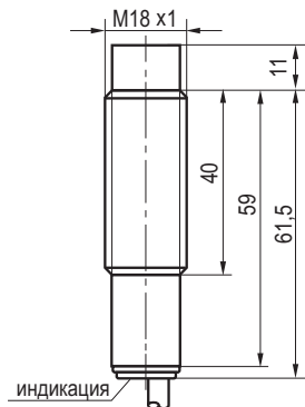
Габаритный чертеж
