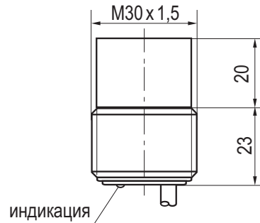
Габаритный чертеж
