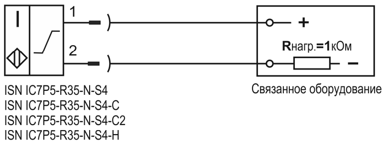
Схема подключения к оборудованию
