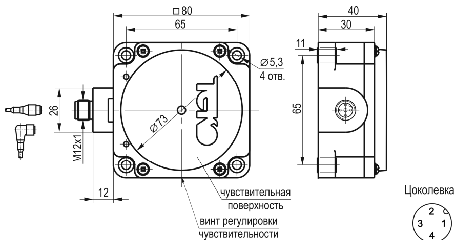
Габаритный чертеж
