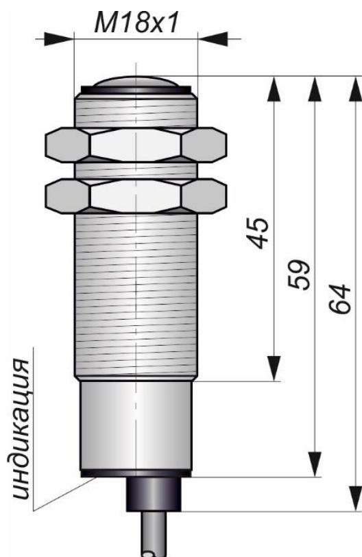
Габаритный чертеж
