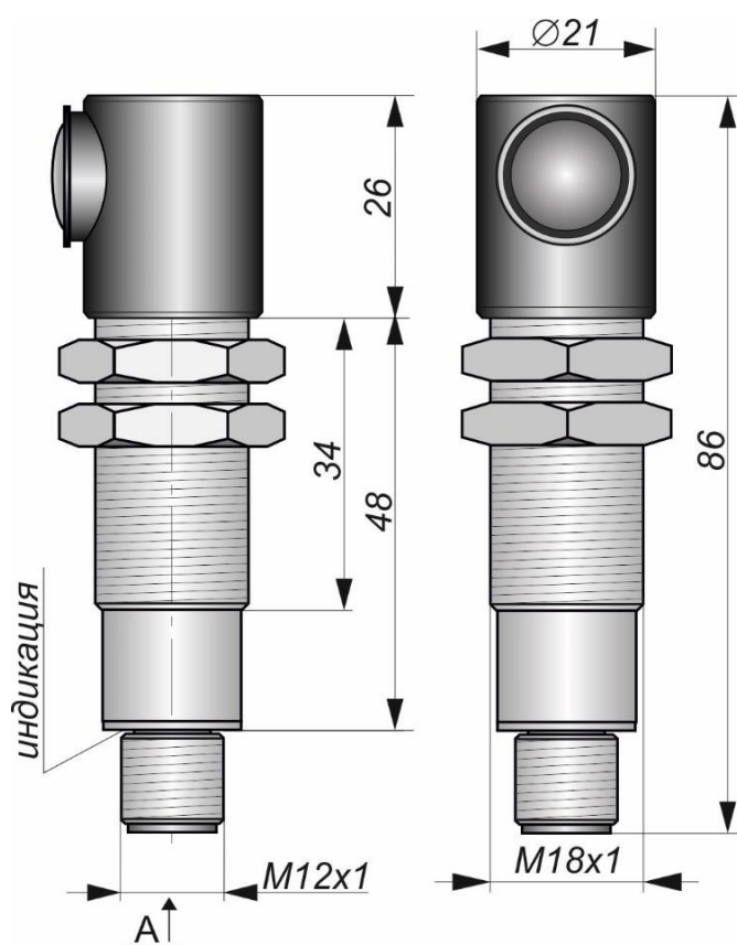
Габаритный чертеж
