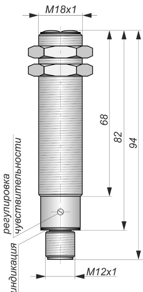
Габаритный чертеж
