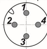
Цоколевка разъема
