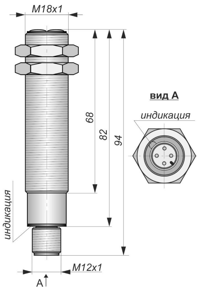
Габаритный чертеж
