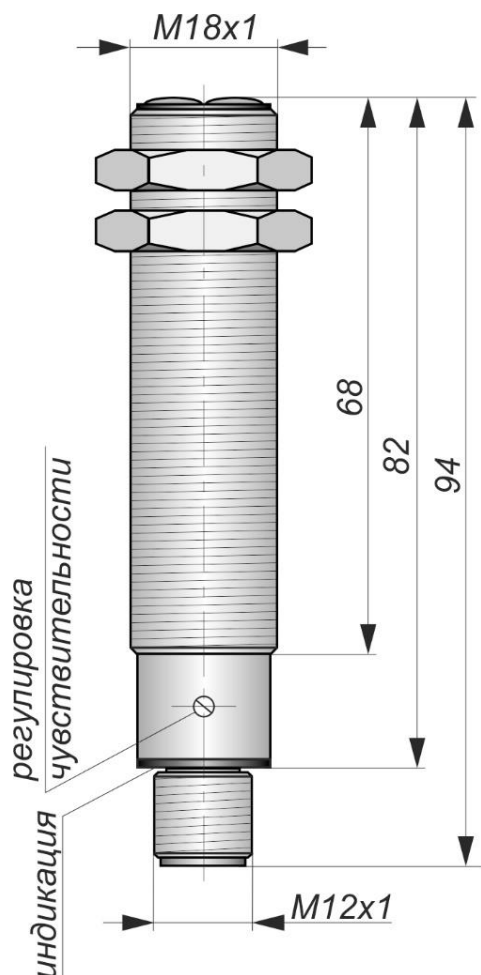
Габаритный чертеж
