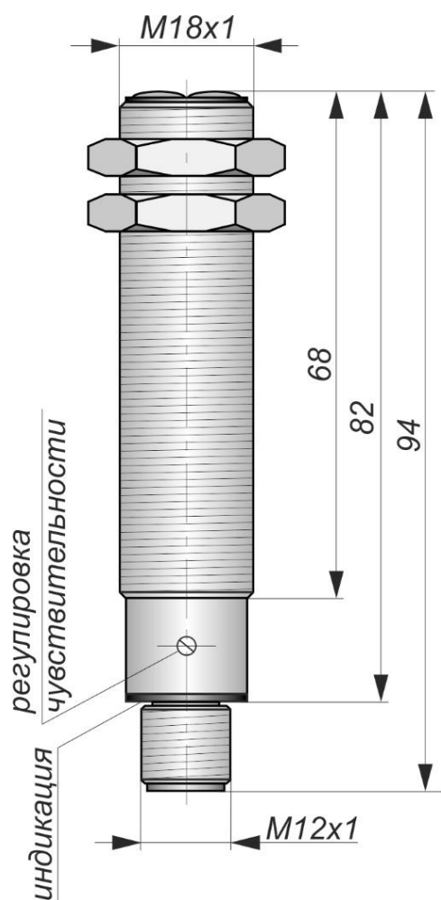
Габаритный чертеж
