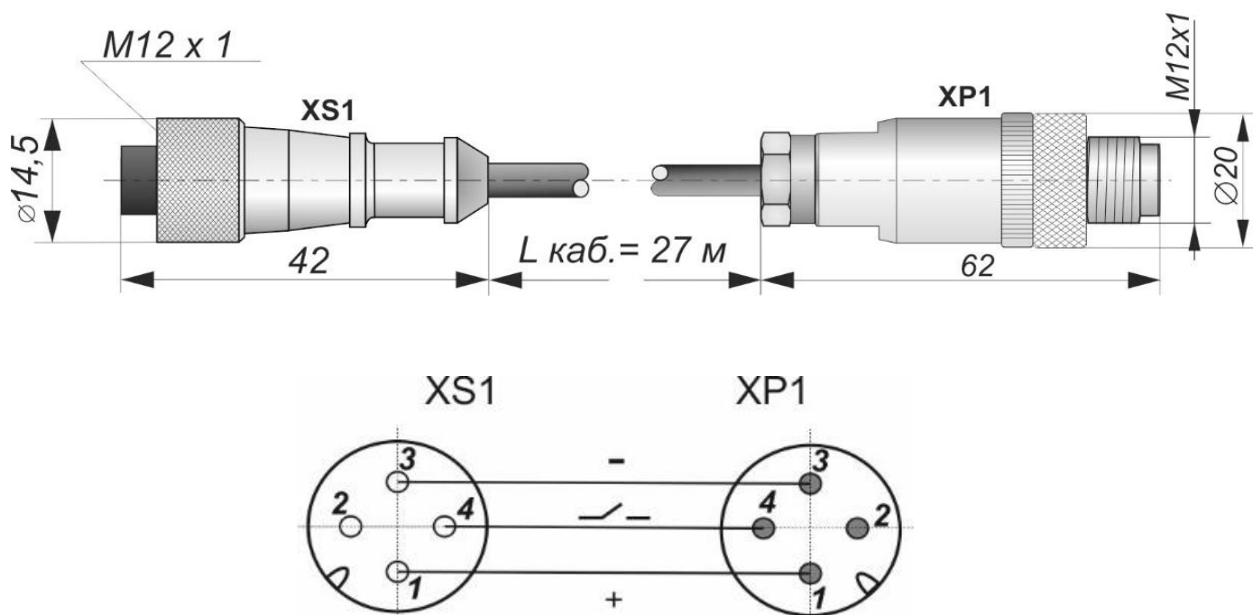
Габаритный чертеж
