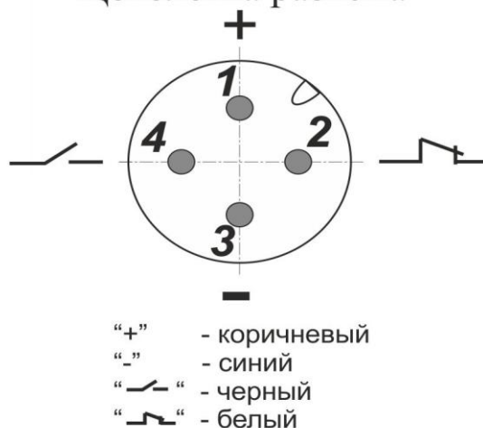
Цоколевка разъема
