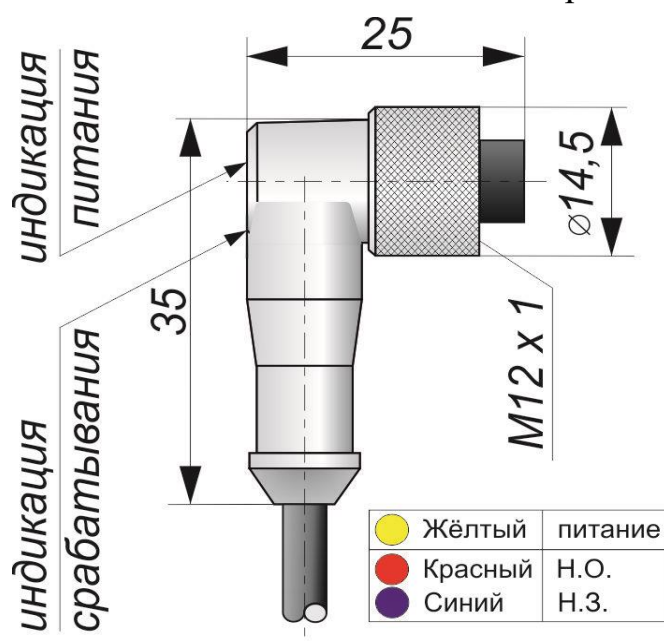
Габаритный чертеж
