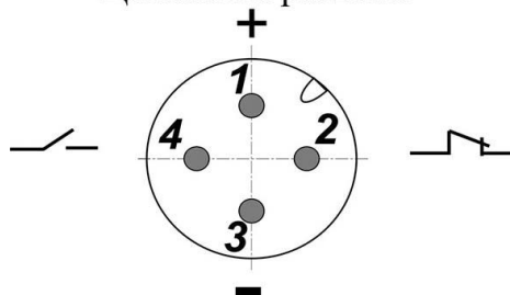
Цоколевка разъема
