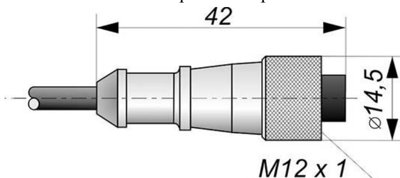
Габаритный чертеж
