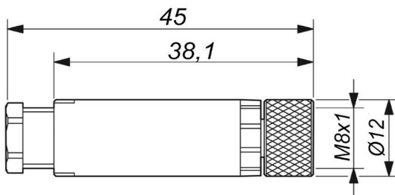
Габаритный чертеж
