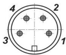
Цоколевка разъема
