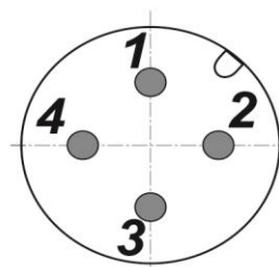
Цоколевка разъема
