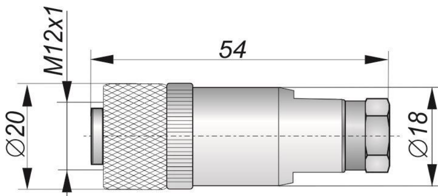
Габаритный чертеж
