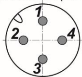
Цоколевка разъема
