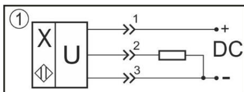
Схема соединения
