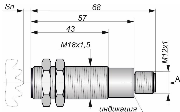
Габаритный чертеж
