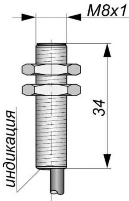
Габаритный чертеж
