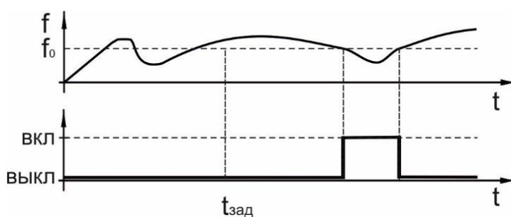
Диаграмма работы датчика
