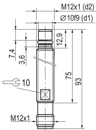
Габаритный чертеж
