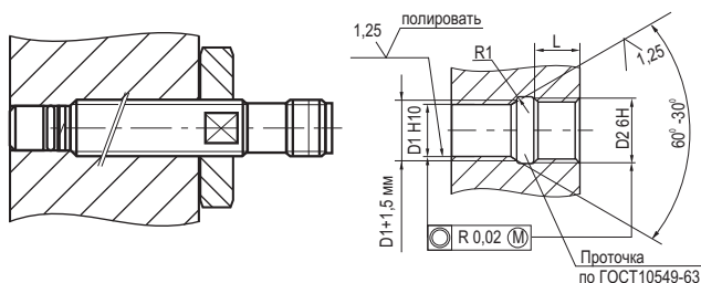
Схема монтажа
