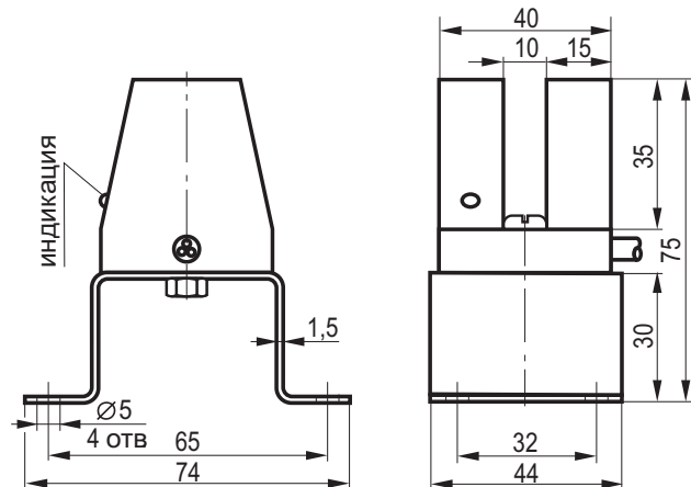
Габаритный чертеж
