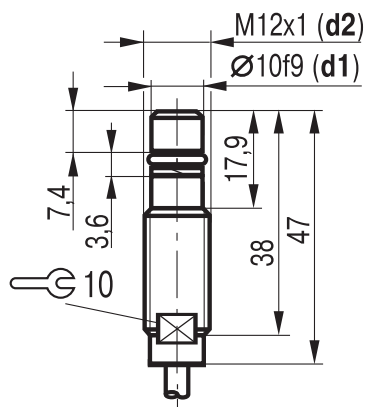
Габаритный чертеж
