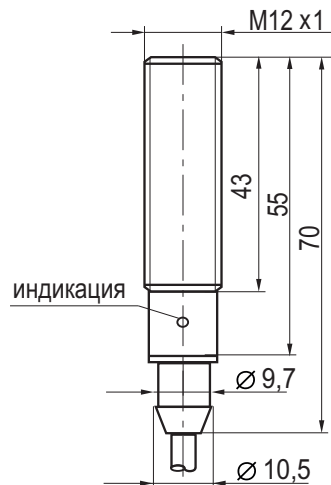
Габаритный чертеж
