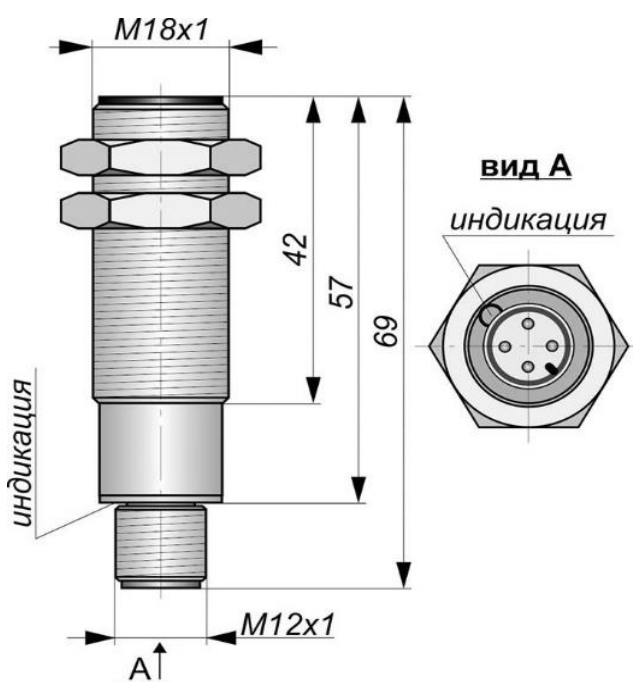
Габаритный чертеж
