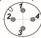
Цоколевка разъема
