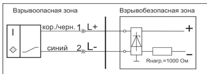
Цоколевка разъема
