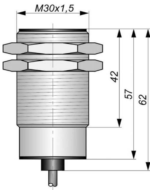
Габаритный чертеж
