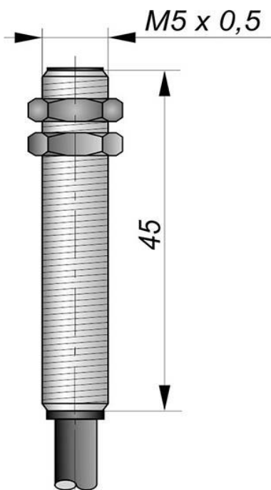
Габаритный чертеж
