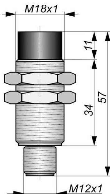
Габаритный чертеж
