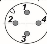
Цоколевка разъема
