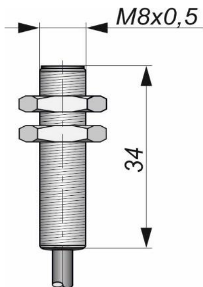
Габаритный чертеж
