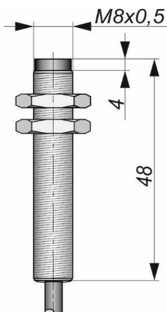
Габаритный чертеж
