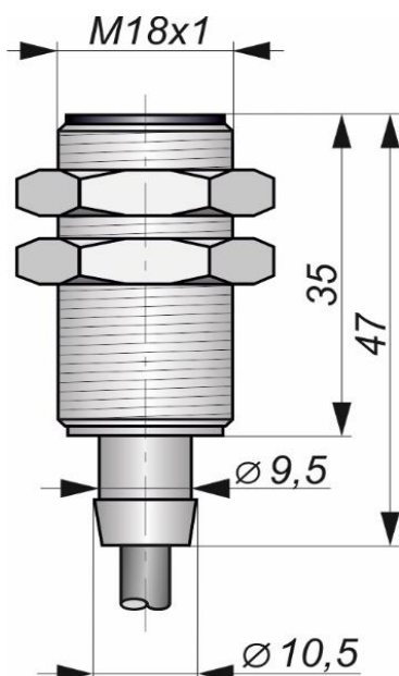
Габаритный чертеж
