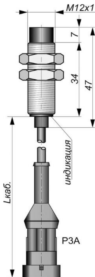
Габаритный чертеж
