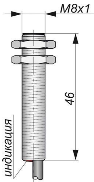
Габаритный чертеж
