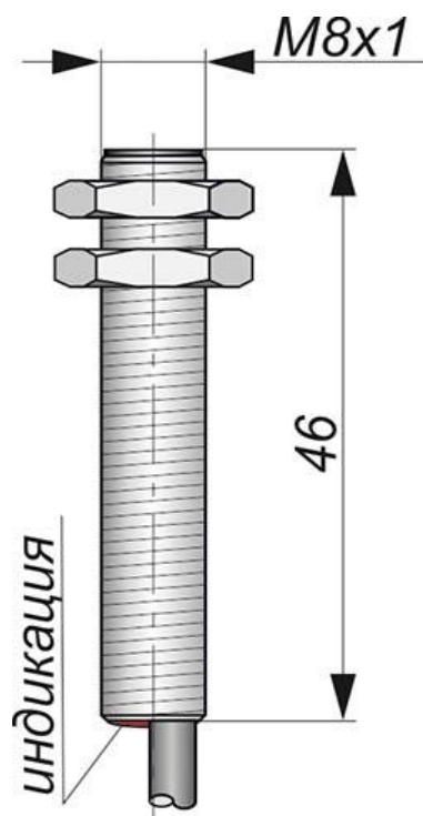
Габаритный чертеж
