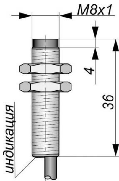
Габаритный чертеж
