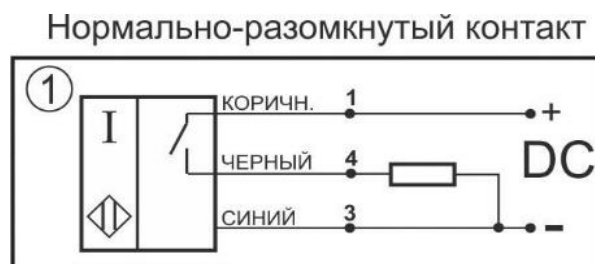
Схема соединения
