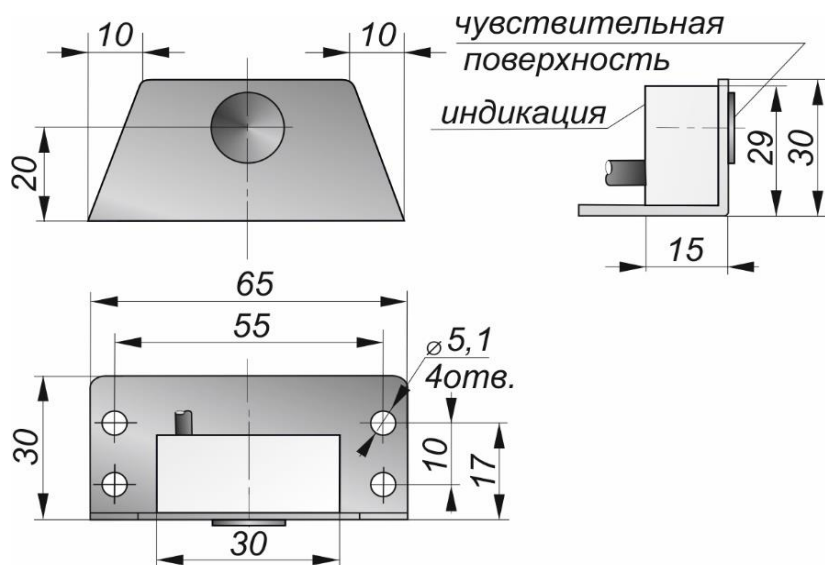
Габаритный чертеж
