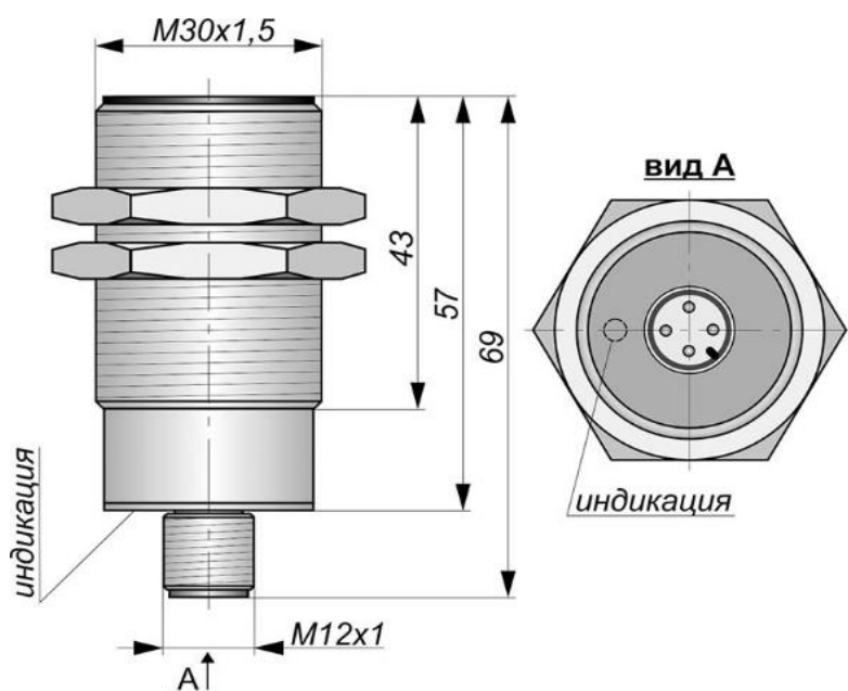
Габаритный чертеж
