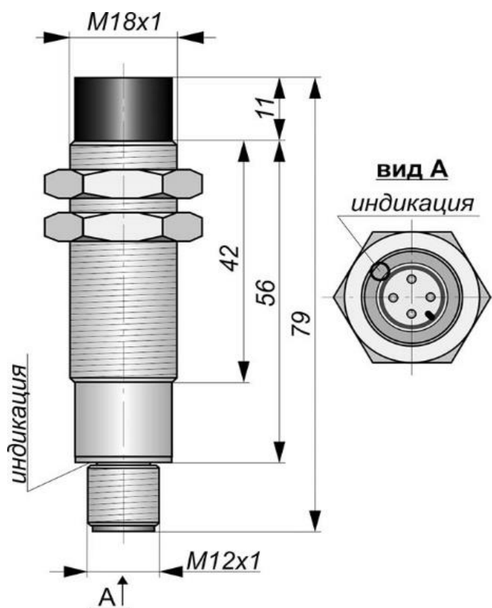
Габаритный чертеж
