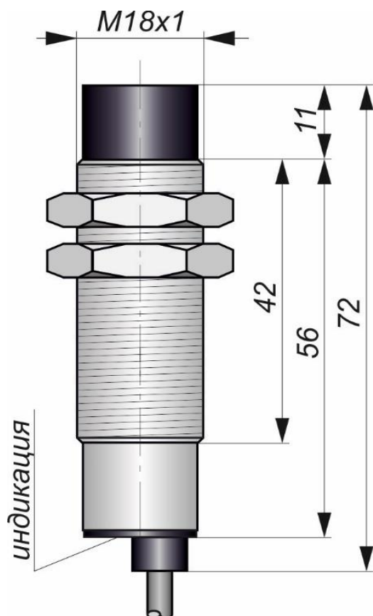
Габаритный чертеж
