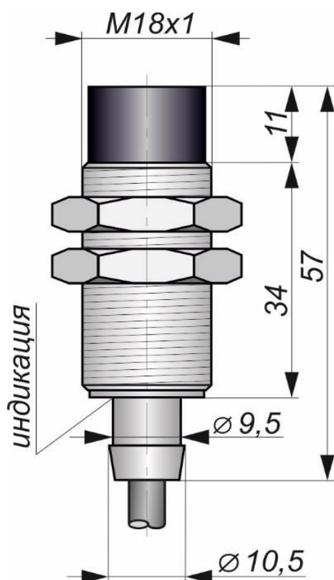
Габаритный чертеж
