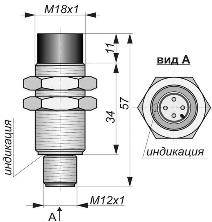
Габаритный чертеж
