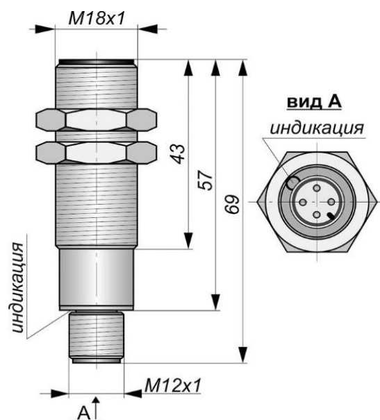
Габаритный чертеж
