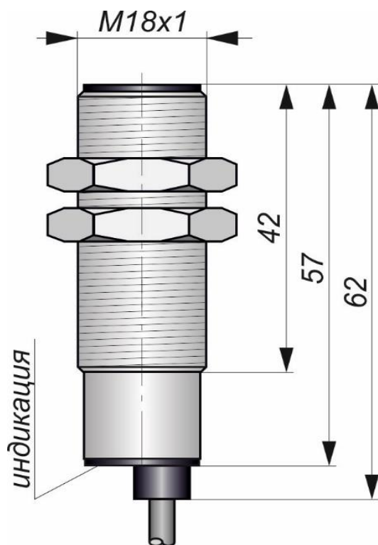
Габаритный чертеж
