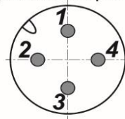
Цоколевка разъема
