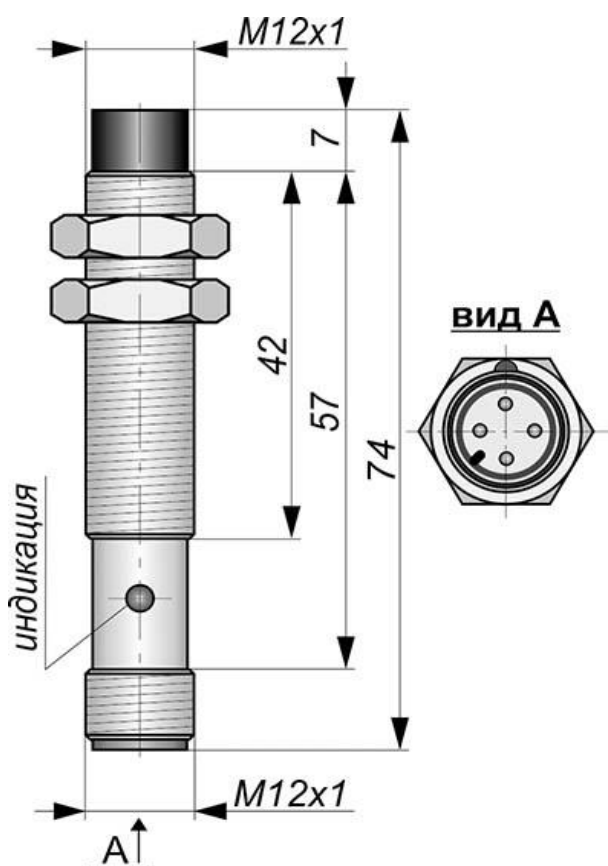
Габаритный чертеж
